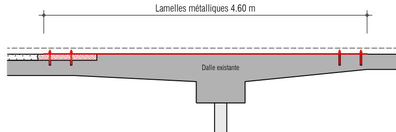
Renforcements de la dalle existante avec lamelles métalliques
