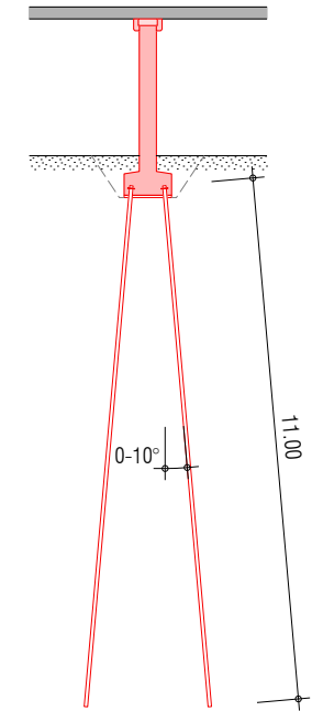
Colonne et micropieux
